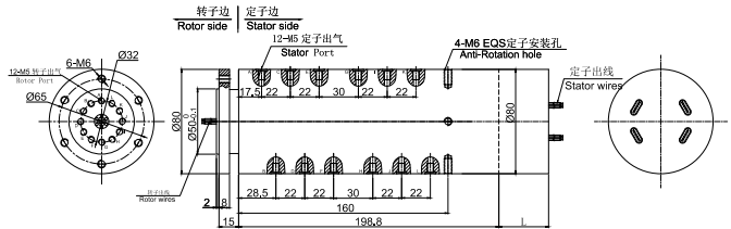
MAPH1200-01气电一体 尺寸图
