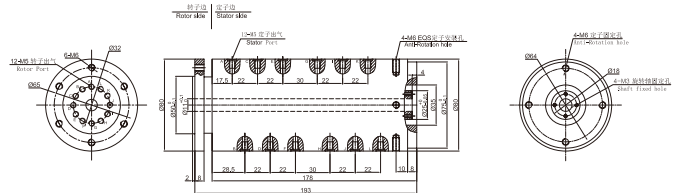
MAPH1200-01气电一体 尺寸图
