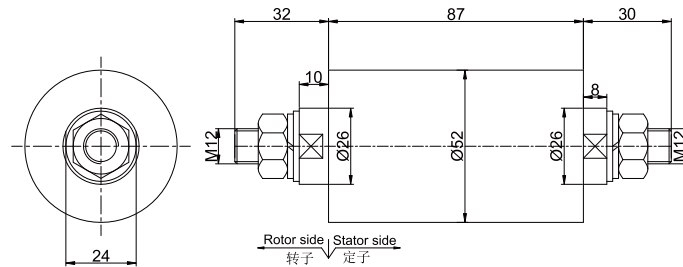
MW5045-P01250 尺寸图
