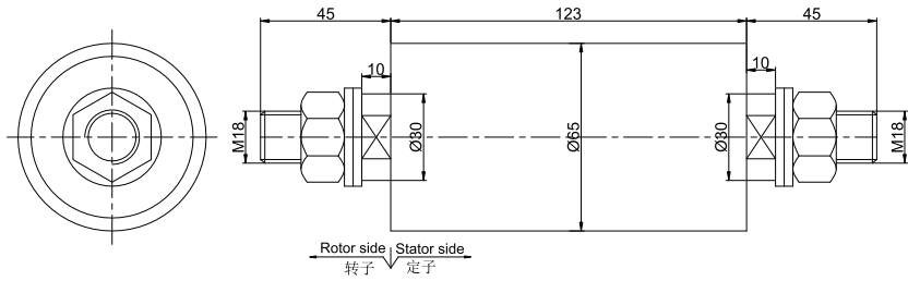
MW5045-P011000 尺寸图
