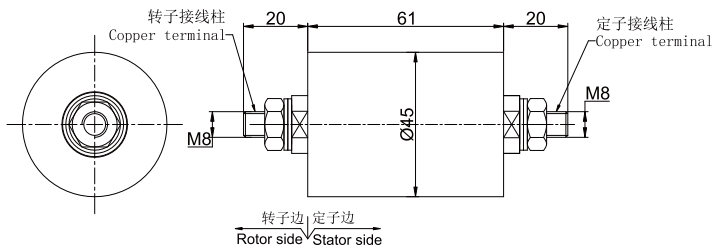
MW5045-P01200 尺寸图
