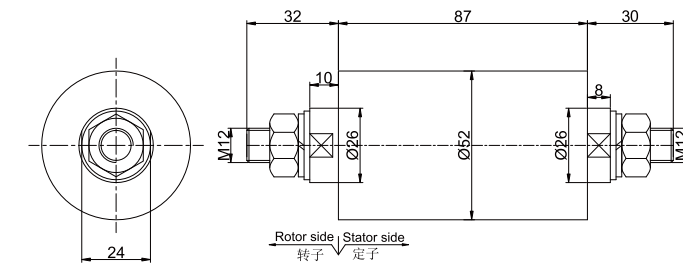
MW5045-P01250 尺寸图
