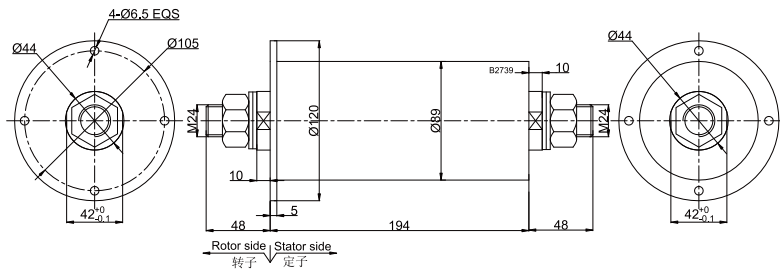
MW5045-P011000 尺寸图
